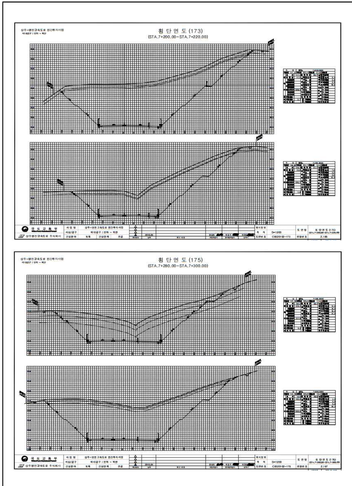
【그림 66-4】 표준횡단면도
